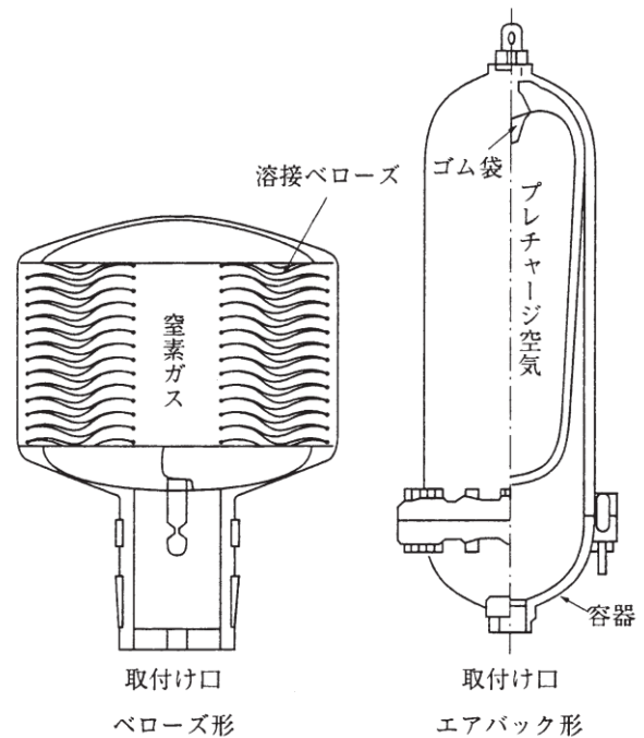
図-6.2.1 水撃防止器具 (給排水・衛生設備の実務の知識)
