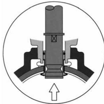
図-6.3.4 管の内面防食
