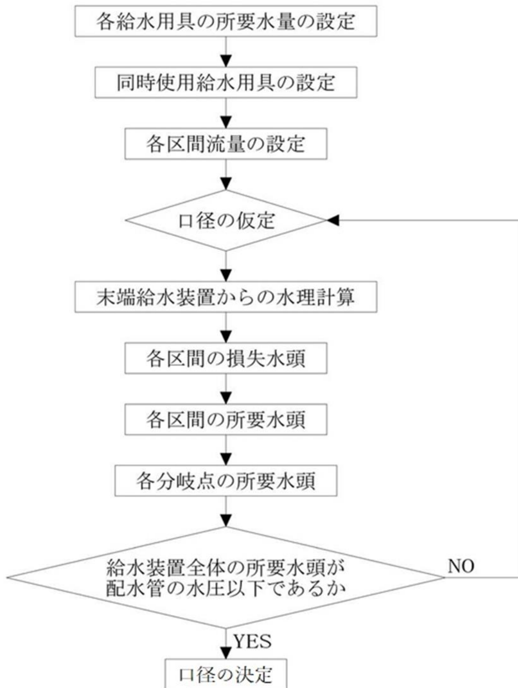
図-2.4.2 口径決定の手順
