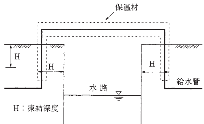
図-6.5.1 水路の防寒措置
