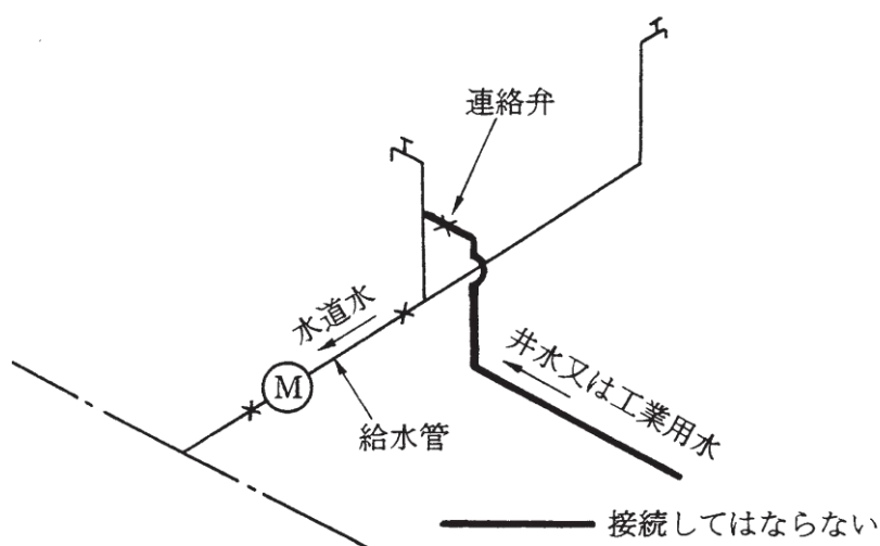
図-6.6.1 接続してはならない配管
