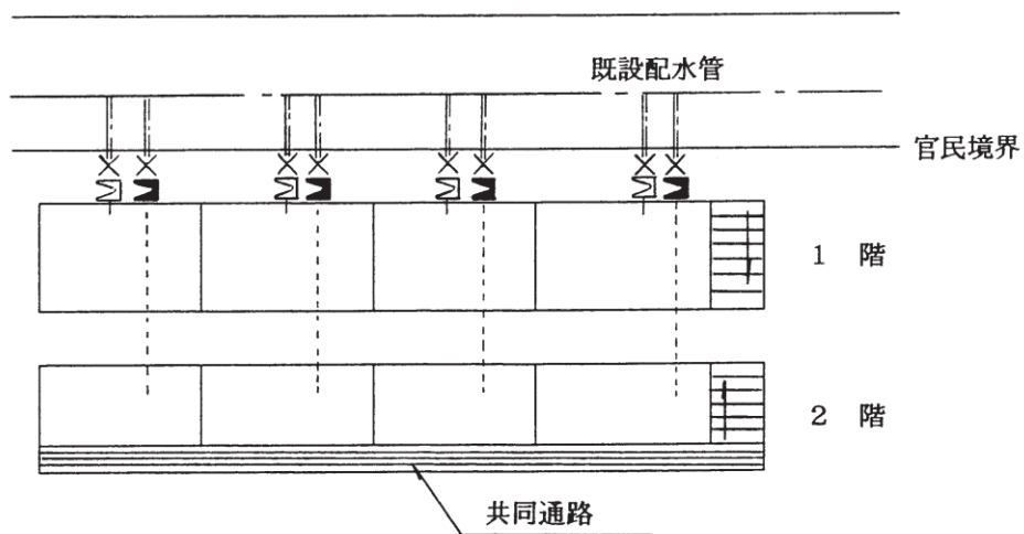
図-5.7.4
