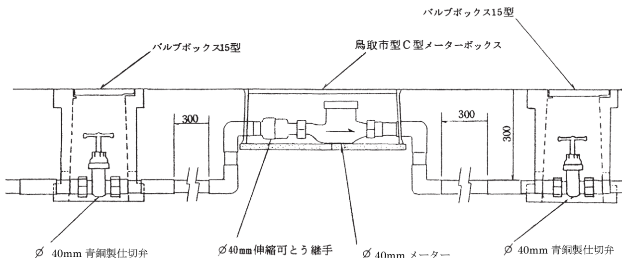
図-5.6.5
