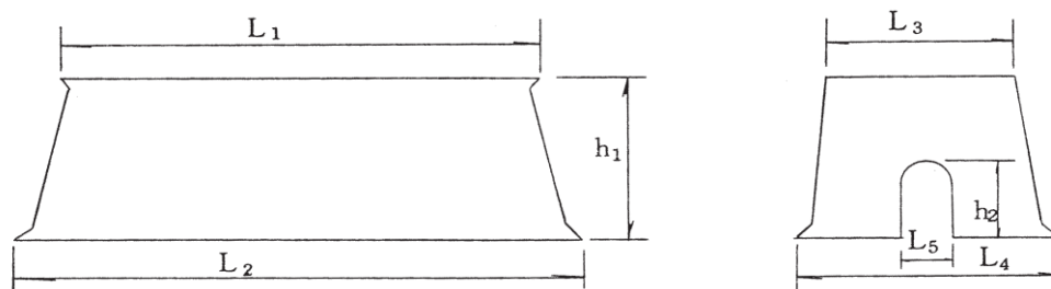
図-5.6.2 鋳鉄製量水器ボックス
