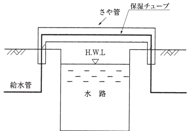
図-6.2.4 上越しの場合
