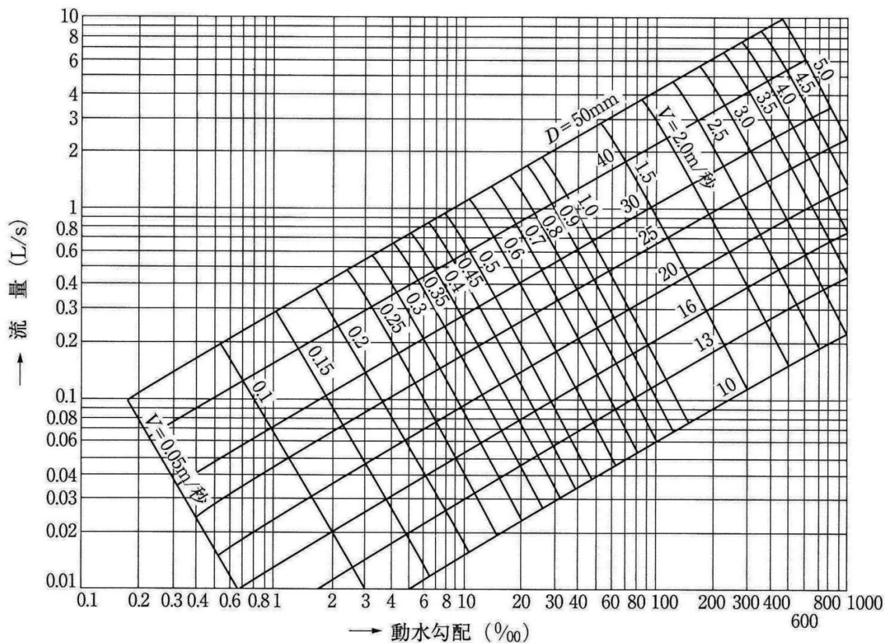
図-2.4.3 ウエストン公式による給水管の流量図
