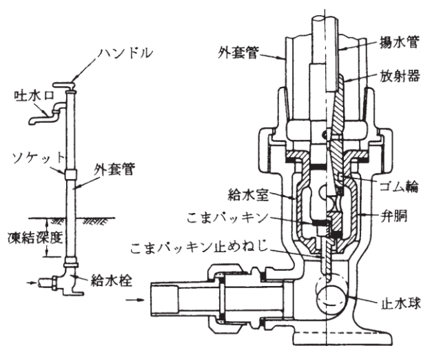
図-6.5.2 内部貯留式不凍給水栓
