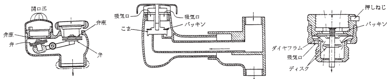
図-6.4.4.2 大気圧式
