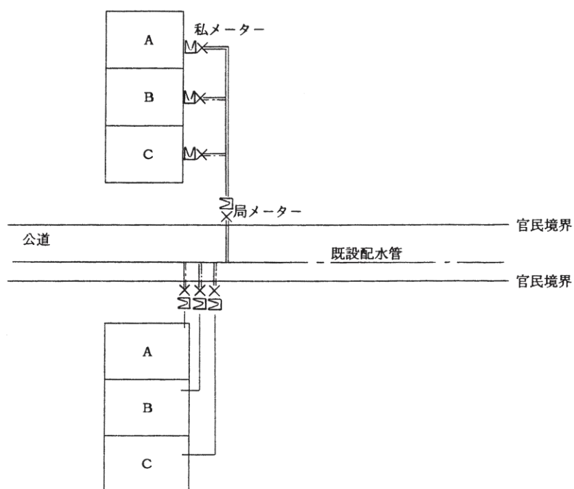
図-5.7.3
