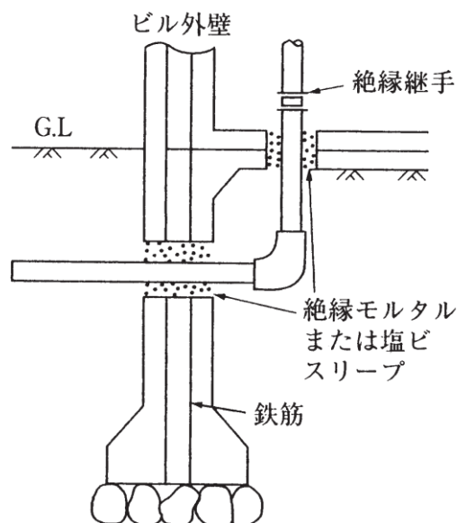
図-6.3.8 ビルに入る配管の絶縁概要図
