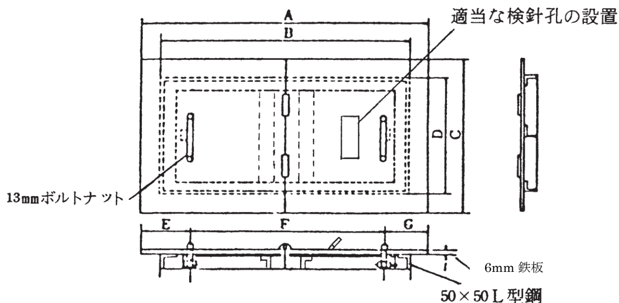
図-5.6.4 大口径メーター鉄蓋寸法図
