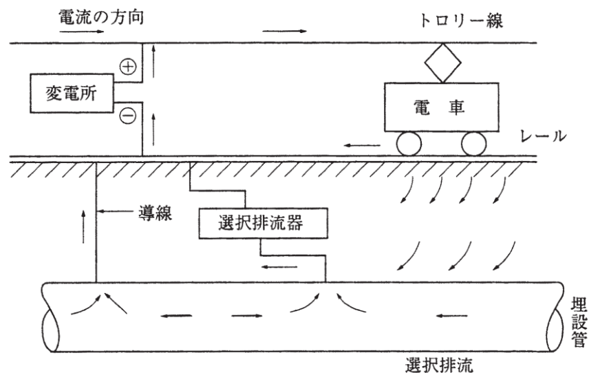
図-6.3.7 選択排流法
