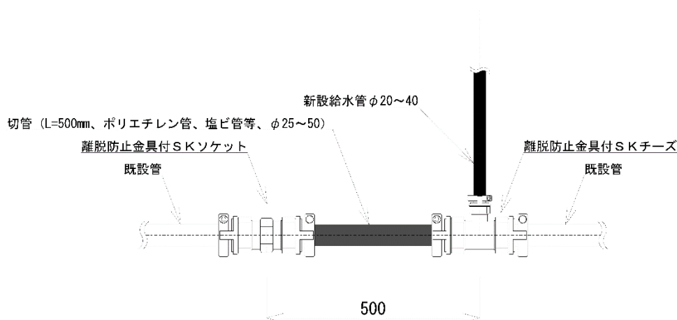
図-5.2.1 配水管からの給水管分岐方法
