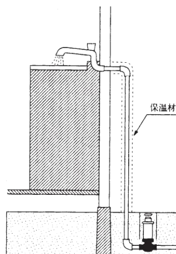
图-6.5.5 屋外操作型水拔栓
