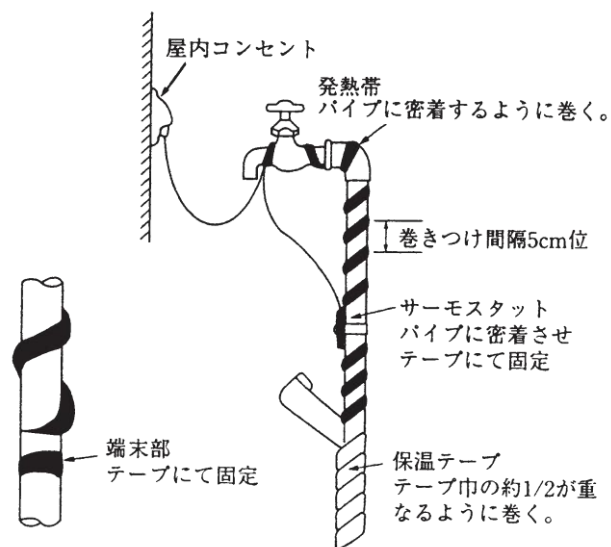
図-6.5.10 加温式凍結防止器
