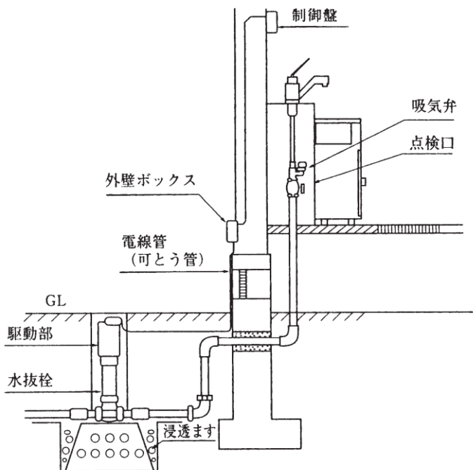
図-6.5.6 屋内操作型水抜栓
