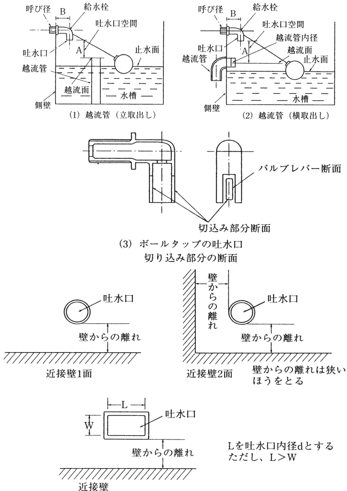
図-6.4.1.2 水槽等の場合
