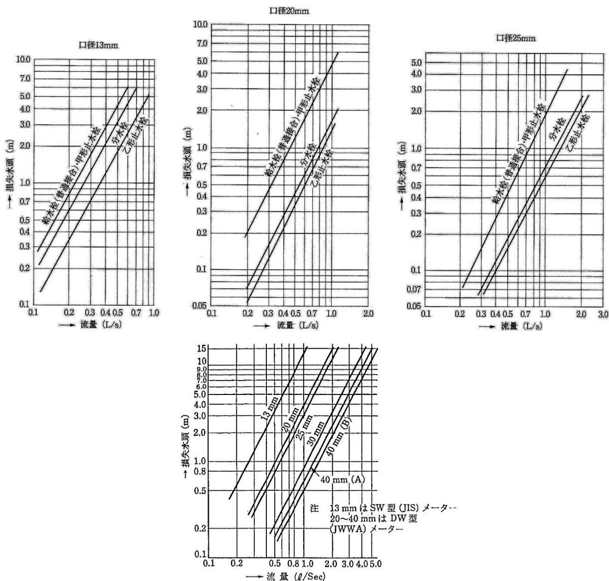
図-2.4.4 各種給水用具の標準使用水量に対応する損失水頭
