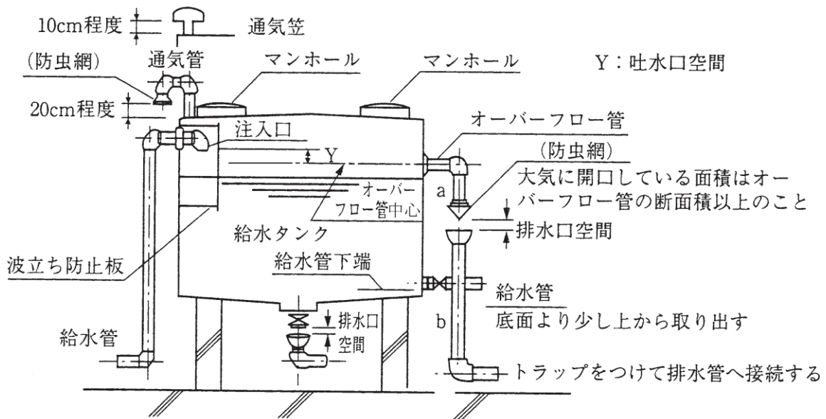
図-6.2.2 受水槽の波立ち防止板
