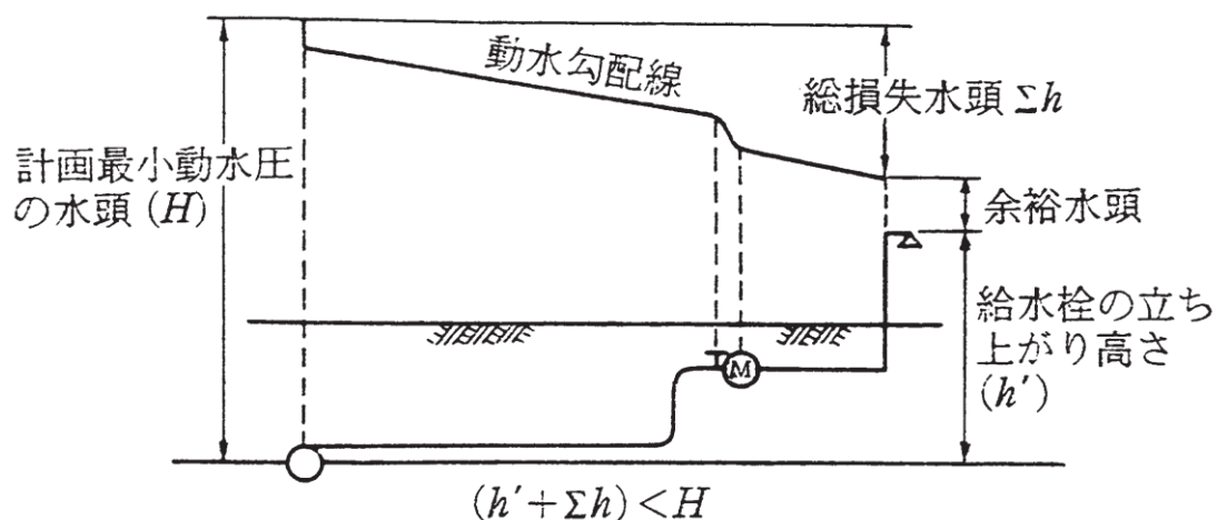
図-2.4.1 動水勾配線図
