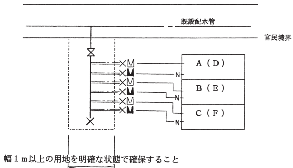
図-5.7.6
