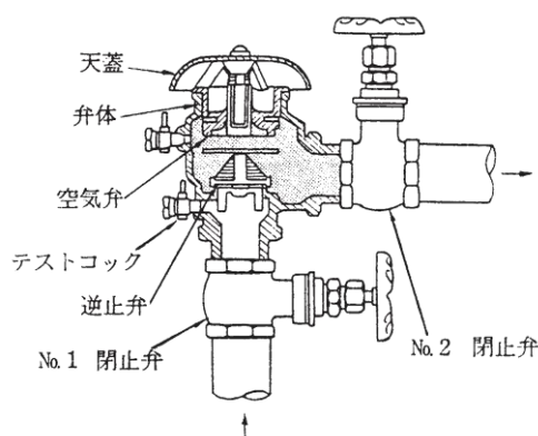
図-6.4.4.1 圧力式
