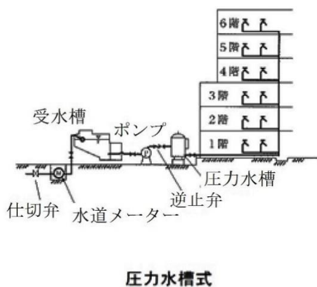
図-2.2.1 給水方式の例
