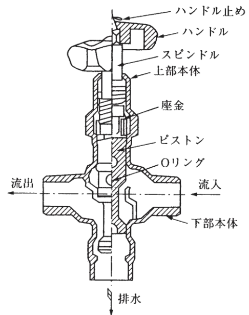
図-6.5.9 水抜きバルブ
