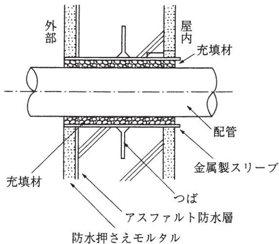
図-6.2.3 配管スリーブの設置
