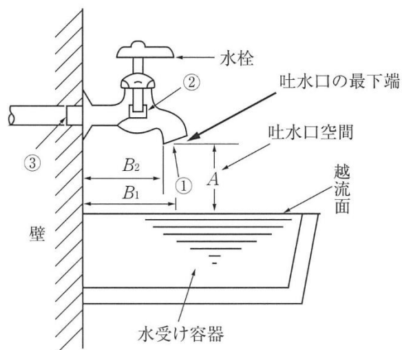
図-6.4.1.1 洗面器等の場合
