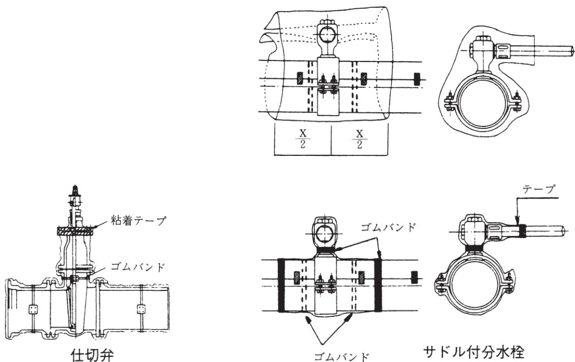
図-6.3.2 サドル付分水栓等の外面防食
