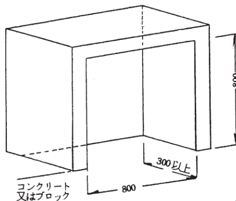
図-5.6.1
