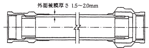
図-6.3.6 電氣的絶縁継手
