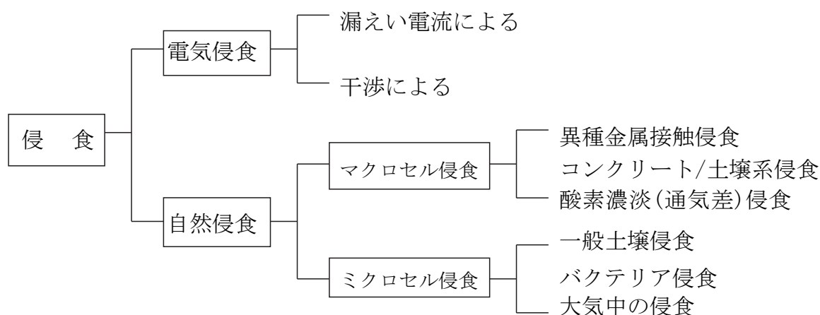
図-6.3.1 金属管の侵食の分類(「給水装置工事技術指針」本編)
